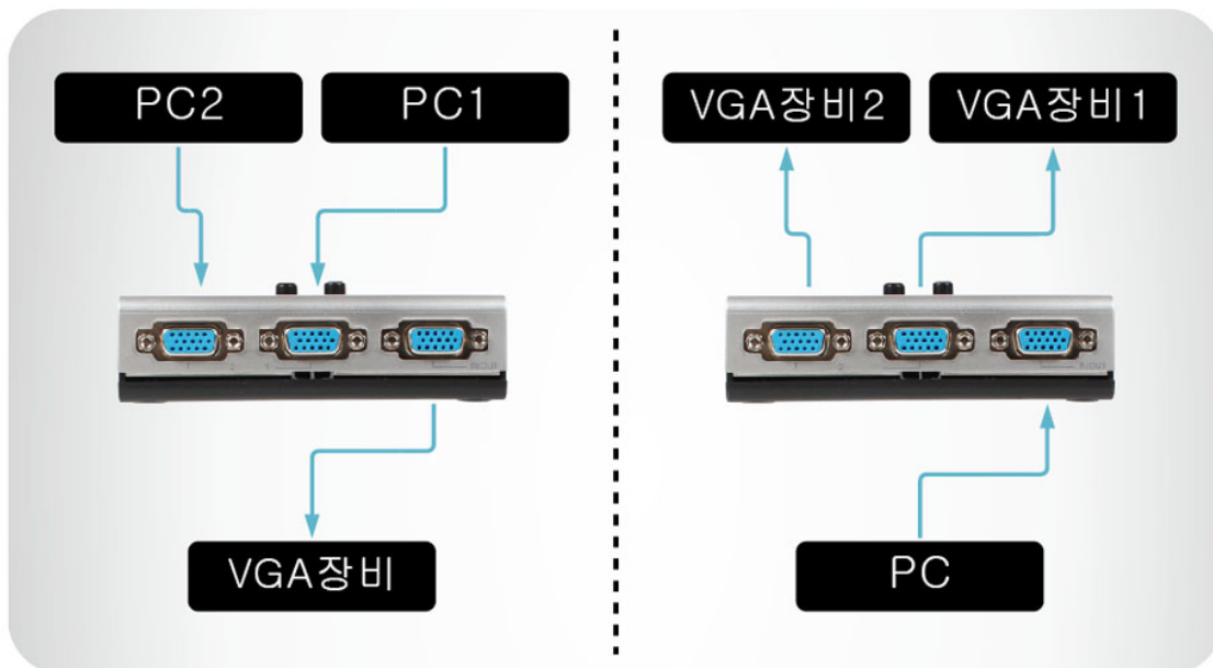
<NM-SS21 제품 연결도>
